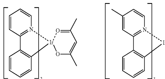
Ir(ppy) 2 (acac)
