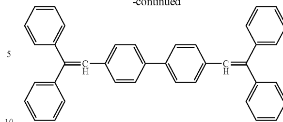
DPVBi
