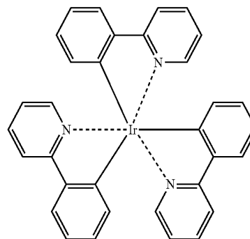
Ir(ppy) 3
