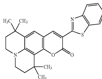
C545T
