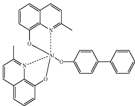
BALq
